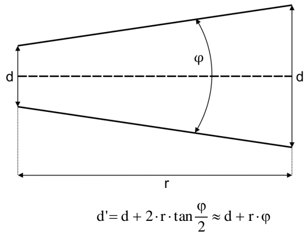
Abb. A2.7 Aufweitung eines Laserstrahls
