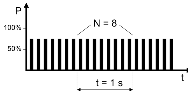
Abb. A2.3 Impulsfolgefrequenz für einen regelmäßig gepulsten Laser mit f_P = 8 Hz
