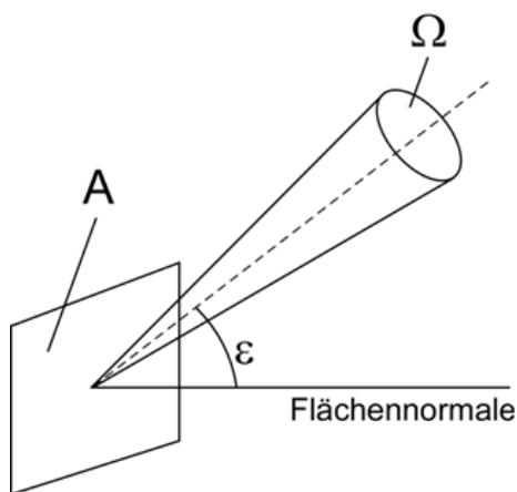
Abb. 2 Strahldichte L unter einem Winkel \varepsilon
